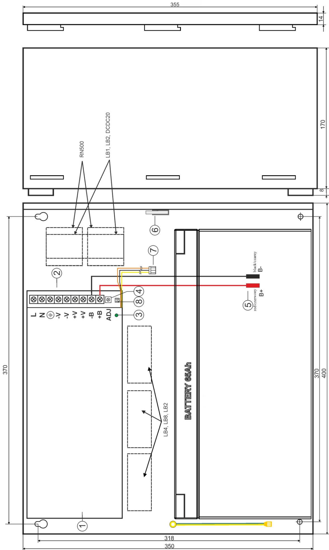
Rys.2. Widok zasilacza.
